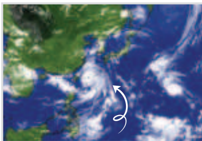
Inçizim satelitor i Tajfunit
